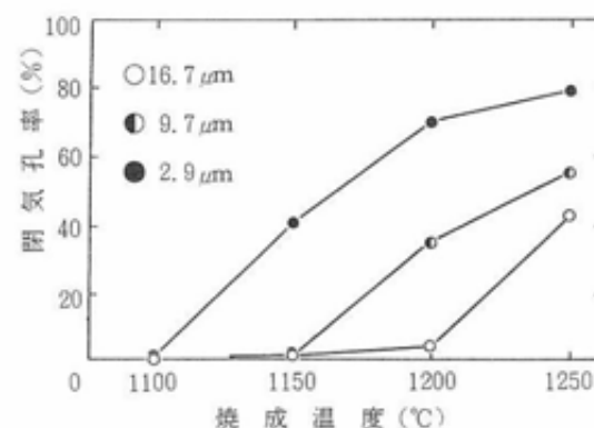
図7 さば発泡体の閉気孔率と焼成温度の関係
