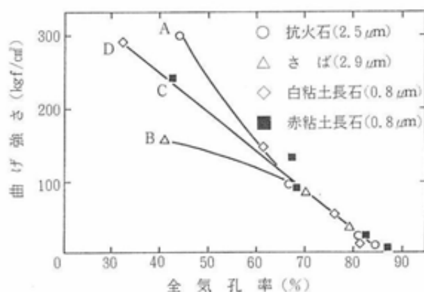
図13 各種発泡体の曲げ強さの比較
