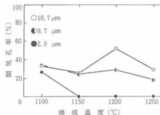
図6 さば発泡体の開気孔率と焼成温度の関係
