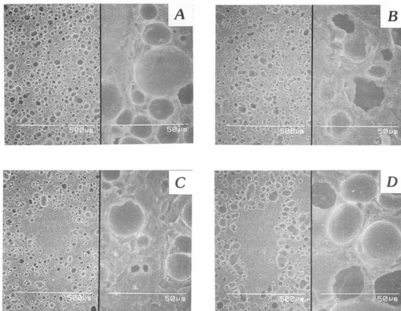
写真2 発泡体断面の電子顕微鏡写真
