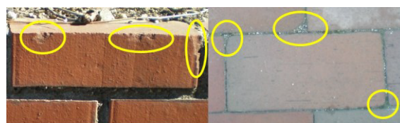
図 2 施工済みれんがの縁・角部の状態 (15 年前後経過、左:花壇、右:歩道)
