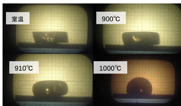
図 2 PDP 廃ガラスの高温加熱顕微鏡像
