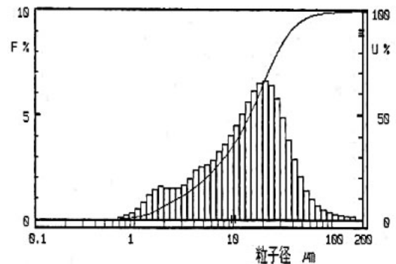
図6 ボールミル粉砕後の PDP 廃ガラスの粒度
