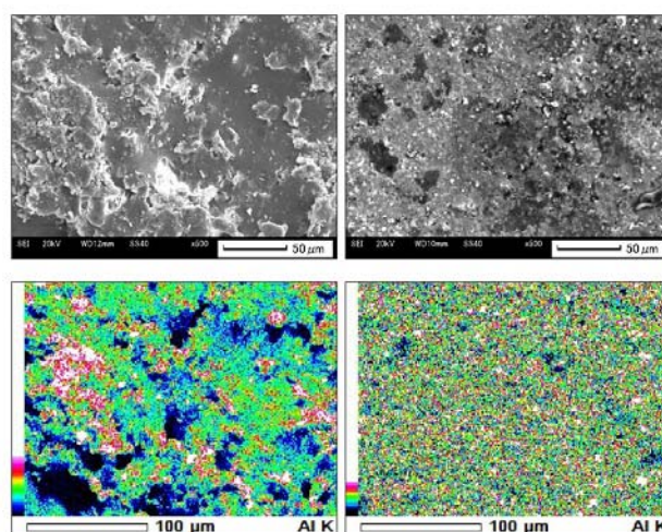
図 9 SEM 像（上）及び Al マッピング像（下） 左：タイル A 右：タイル B
