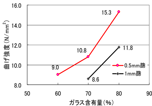
図5 テストピースの曲げ強度
