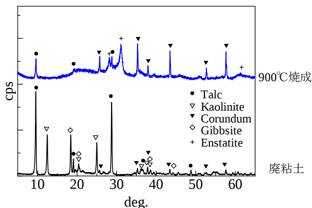
図 4 廃粘土及びその焼成物の X 線回折パターン
