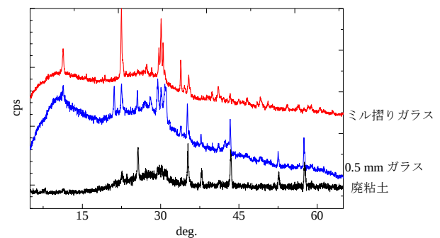
図7 テストピースの X 線回折パターン
