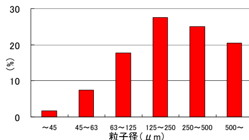
図 3 粉砕後の PDP 廃ガラス粒度分布
