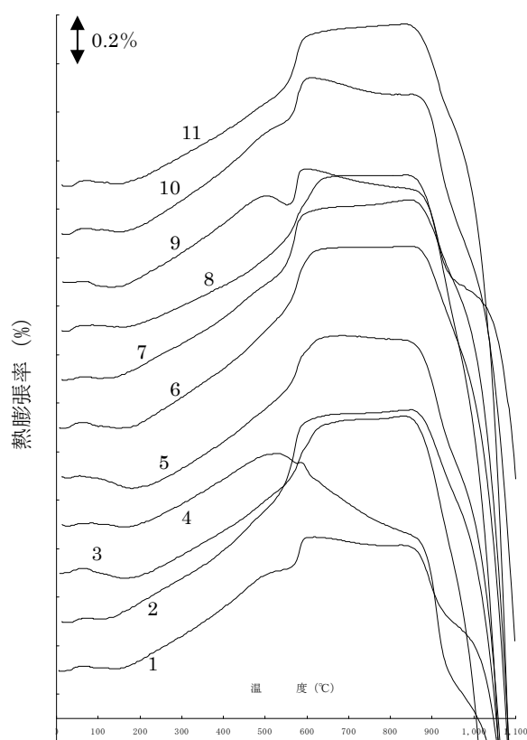
図2 試料 No.1～11 の熱膨張曲線
