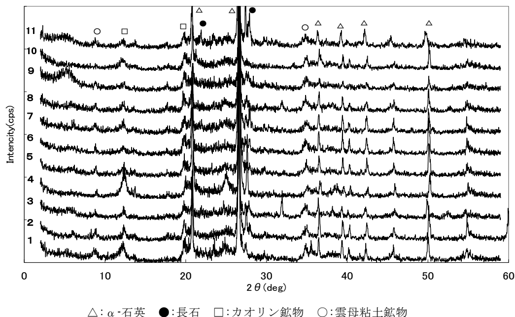
図 1 X 線回折図
