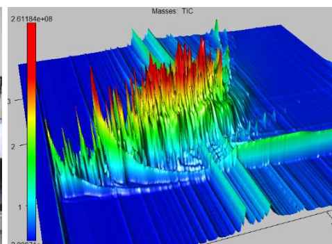
取得した 2 次元クロマトグラフ
